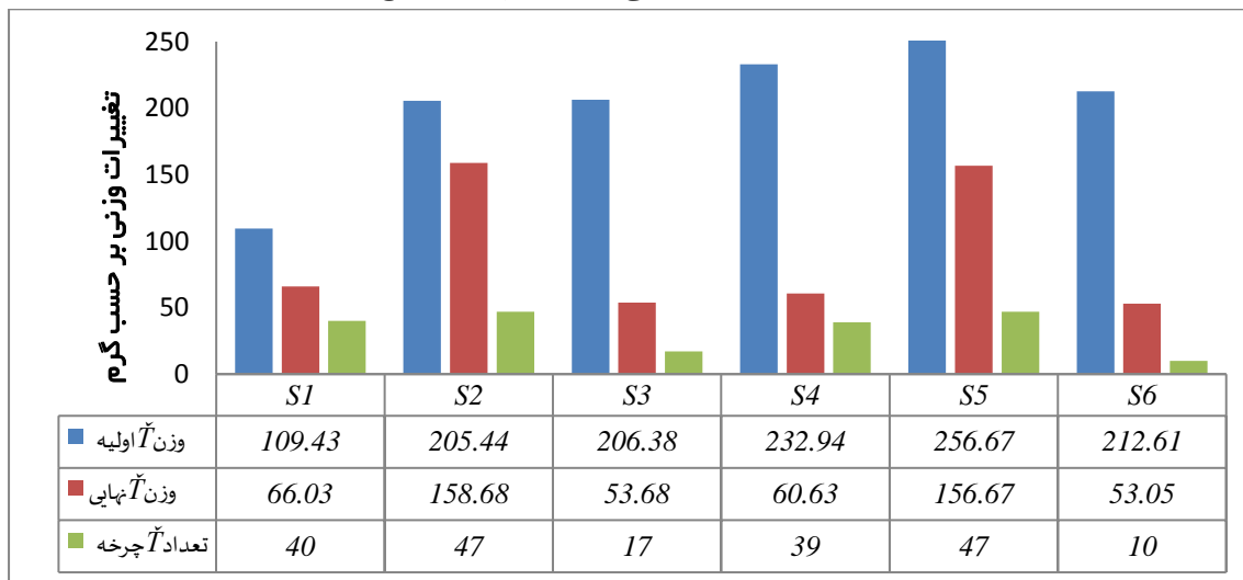
تصویر ۸. نمودار نتایج چرخه پیرسازی شکستگی نمک (مأخذ: نگارندگان)
