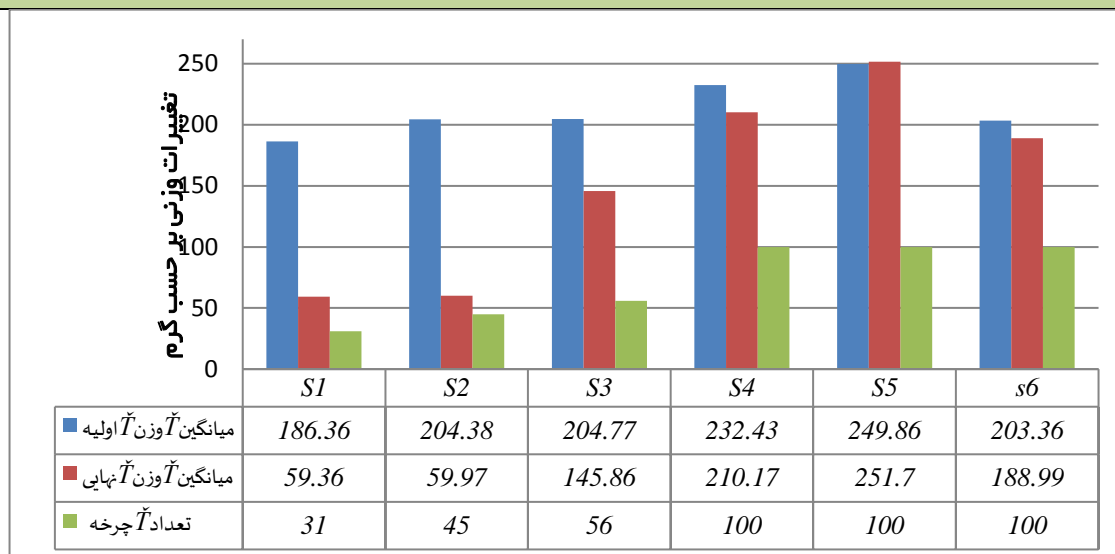
تصویر ۶- نمودار نتایج آزمون چرخه تر و خشک شدن متوالی (مأخذ: نگارندگان)
