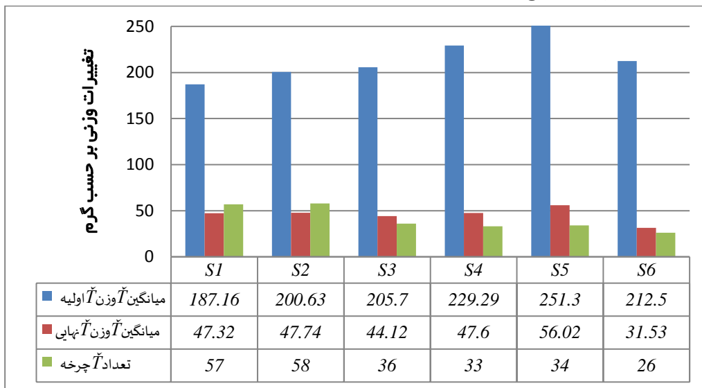
تصویر ۷. نمودار نتایج آزمون پیرسازی انجماد و یخ‌گشایی (مأخذ: نگارندگان)
