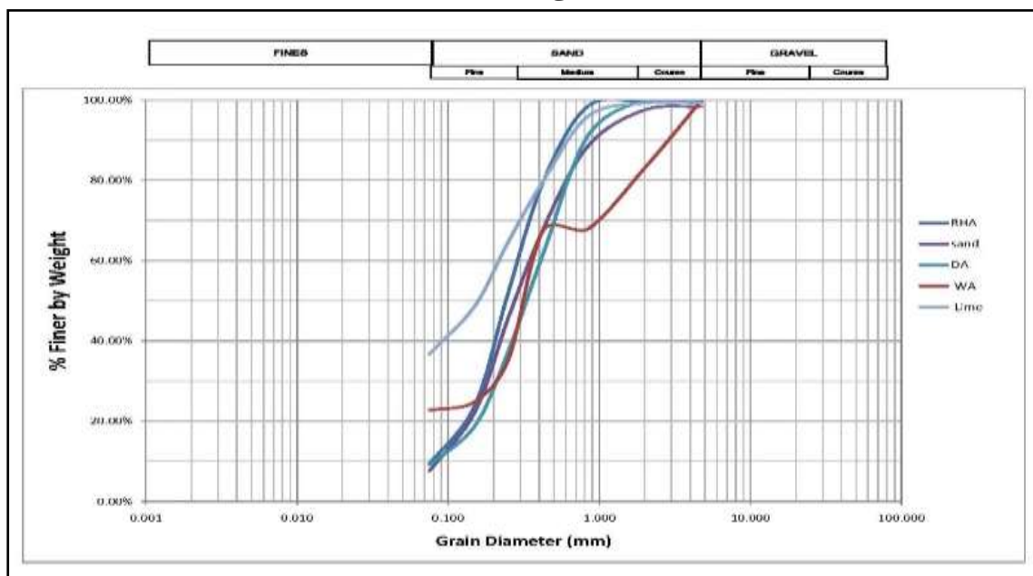
تصویر ۵. نمودار دانه‌بندی مصالح به کار رفته در نمونه‌های ملات (مأخذ: نگارندگان)
