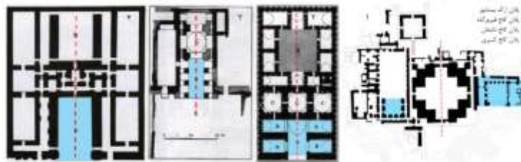
تصویر ۱: مقایسه شکل ایوان در چند بنای ساسانی؛ منبع پلان ۱، نگارنده براساس نقشه گیرشمن و نقشه پایگاه میراث فرهنگی بیشاپور؛ منبع پلان ۲، ۳ و ۴، (پوپ: ۱۳۸۲، ۵۵، ۶۴ و ۵۸).
