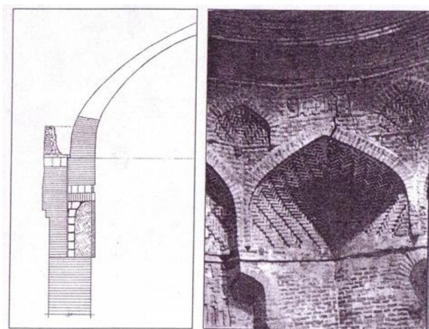
شکل ۸) گوشه‌سازی و شیوه برپایی گنبد امامزاده عقیل (نیک‌زاد و اسفنجاری، ۱۳۸۴)
