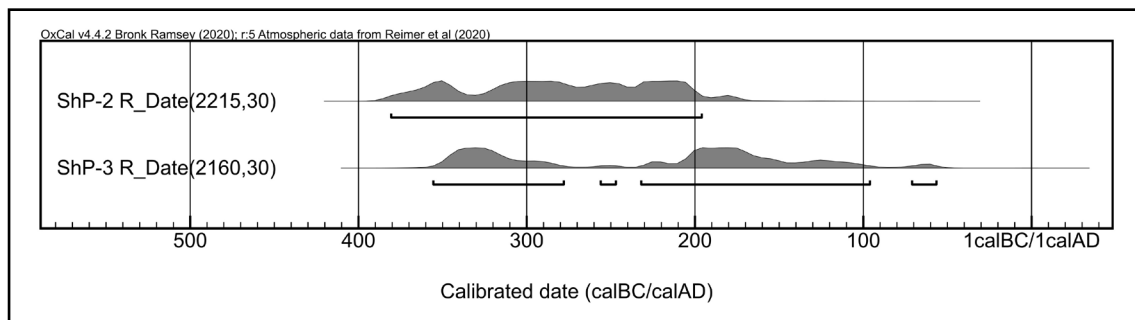
شکل ۴: نتایج تاریخ‌گذاری مطلق دو نمونه زغال از کانتکست‌های ۴ و ۵ در ترانشه استقرار ۷ (نگارندگان، ۱۴۰۴) Fig. 4: Results of C14 analyzing of two charcoal samples from Con. 4 and 5 in Tr. 7, Shahne Poshte (Authors, 2025)
